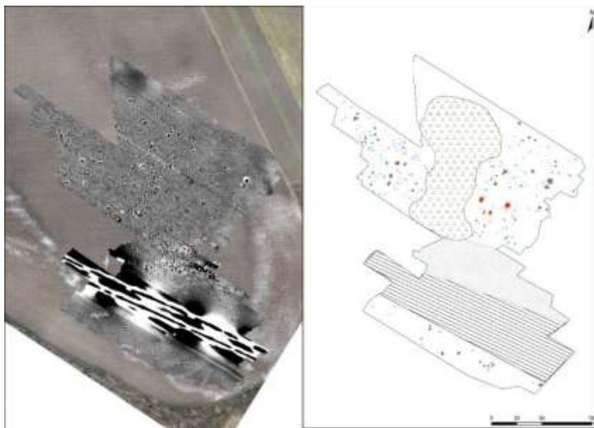
Figura 11. Cartarea geofizică și delimitarea structurilor de interes arheologic din situl de la Topolovățu Mare
